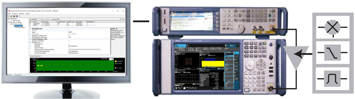
图1. 使用Signal Studio Pro与SP200V系列信号发生器和分析仪的测试配置。
